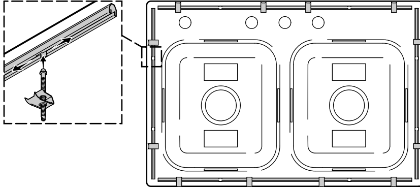
Recommended Clip Placement Emplacement recommandé pour les clips Lugar de instalación recomendado para los clips
